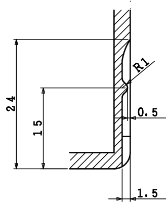
A-A (2:1)
